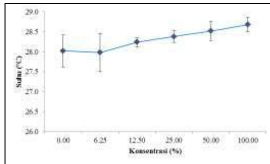
Gambar 3. Pengukuran Suhu pada Uji Pendahuluan
